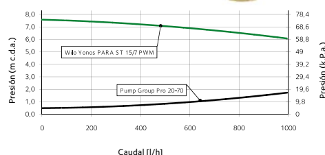
Curva de funcionamiento de la bomba solar 20-70
