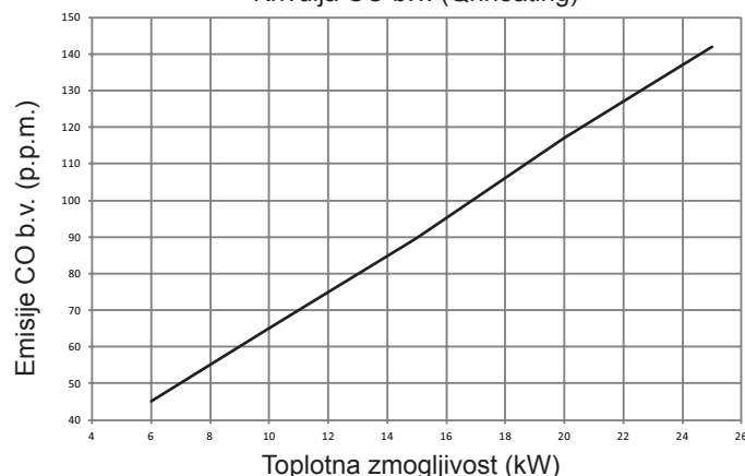
Krivulja CO b.v. (Qnheating)
