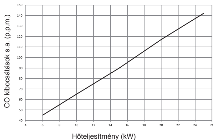
COs.a. görbe (Qnheating)
