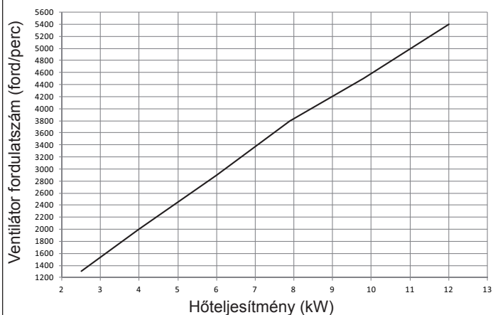
HTG görbe (Qnheating)
