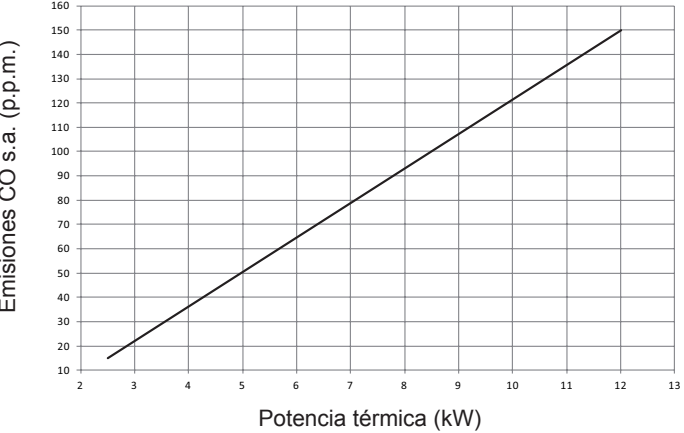
Curva COs.a. (Qn calefacción)
