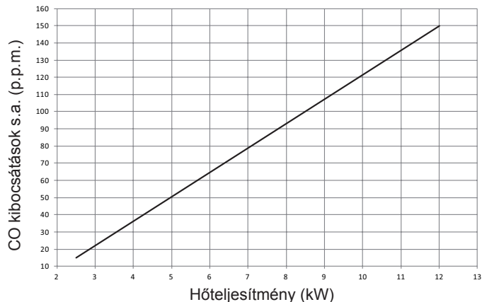
COs.a. görbe (Qnheating)
